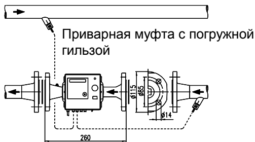
Пример монтажа теплосчетчика с фланцевым соединением
