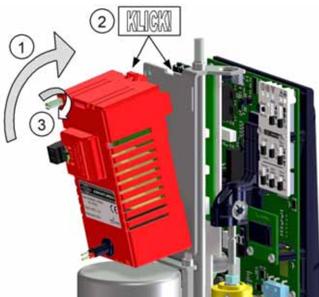
рис. 14: Монтаж и подключение блока питания ARI-PREMIO®-Plus 2G 9 кН с функцией безопасности и ARI-PREMIO®-Plus 2G 25 кН
