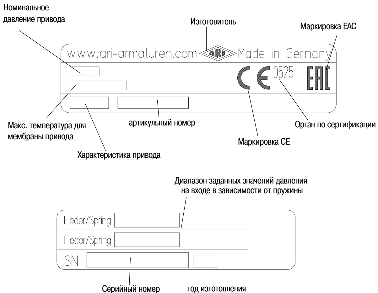
Рис. 3: Привод
