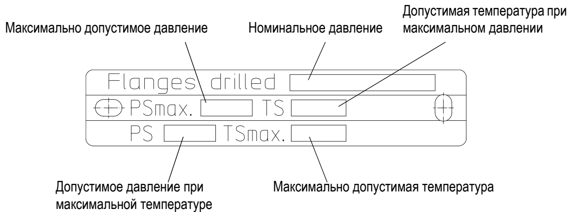
Рис. 4: Фланец
