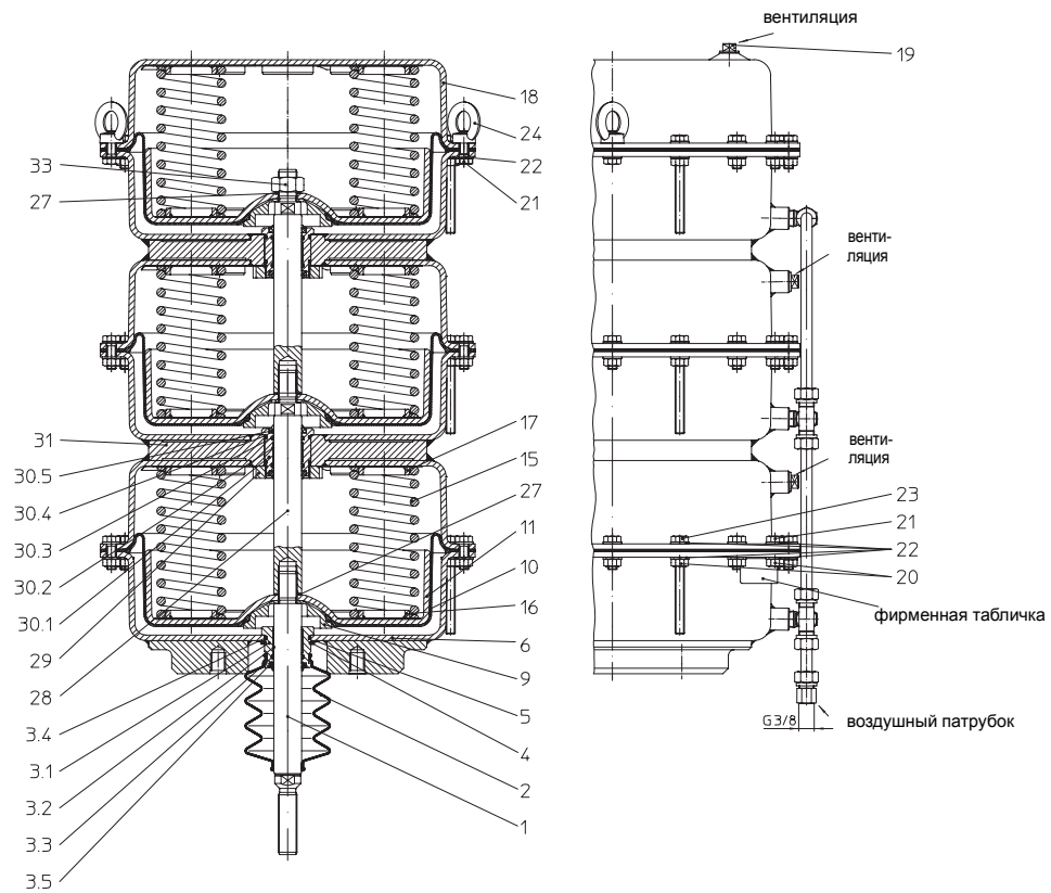
Рис. 5: DP34Tri „шпindelь привода выдвигается за счет силы пружины“
