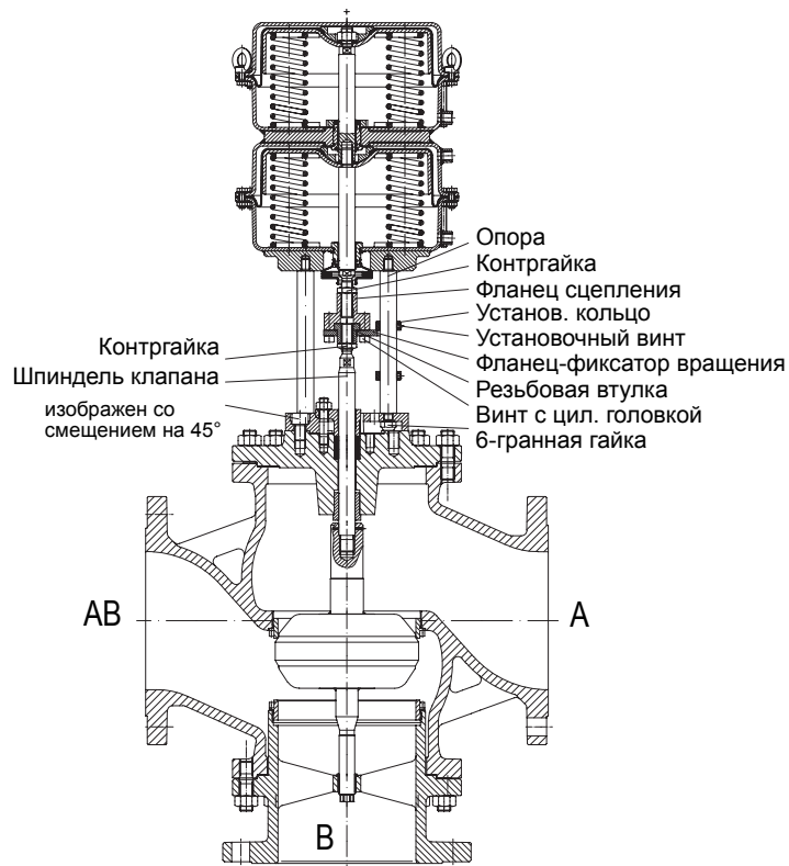
Рис. 11: Пневматический трехходовой сервоклапан в качестве смесителя (проход AB-B) Принцип действия привода: „шпindelь привода втягивается за счет силы пружины“ Пружина закрывает путь A - AB при отказе вспомогательного питания.
