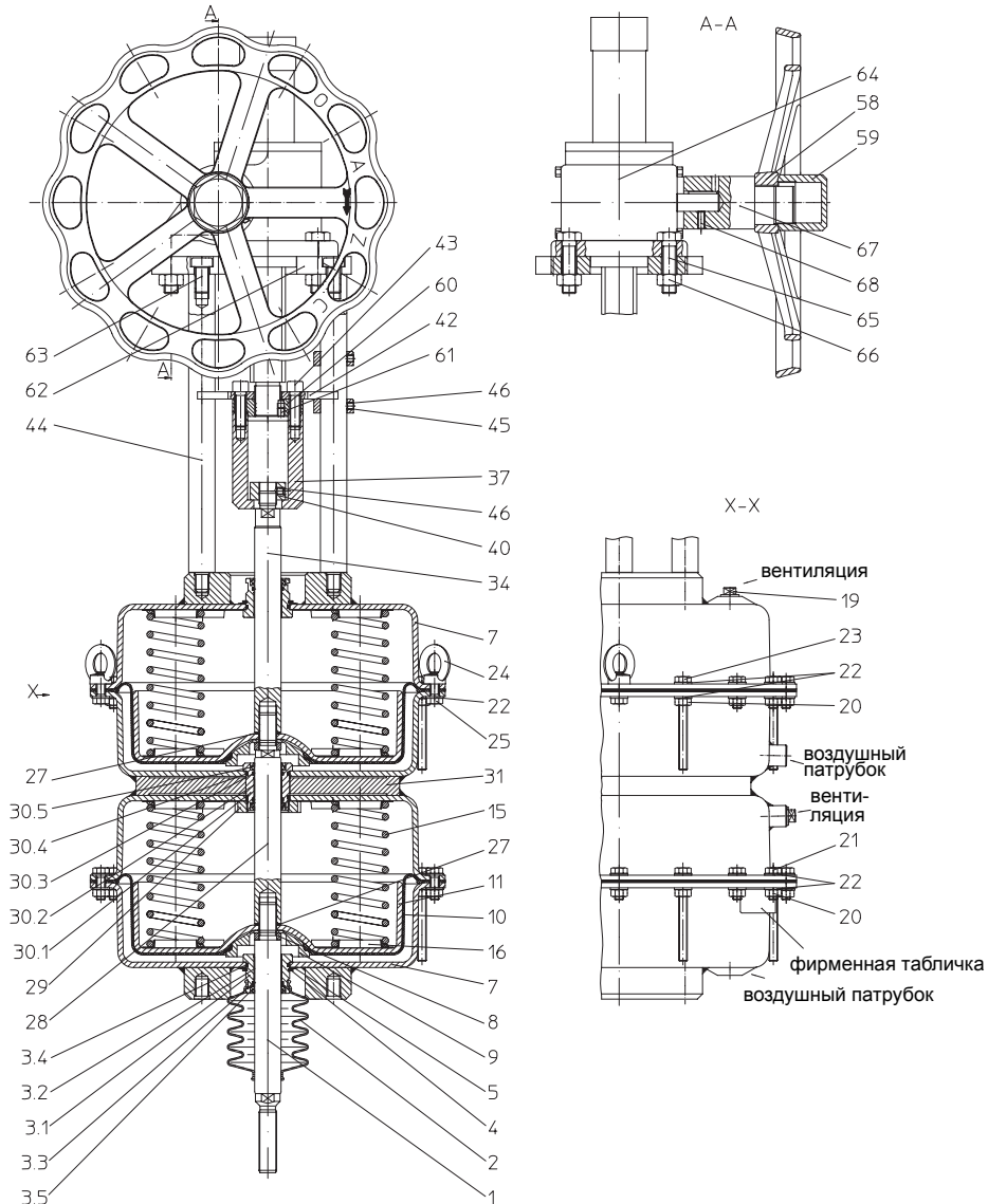
Рис. 2: DP34T „шпindelь привода выдвигается за счет силы пружины“ с аварийным ручным управлением
