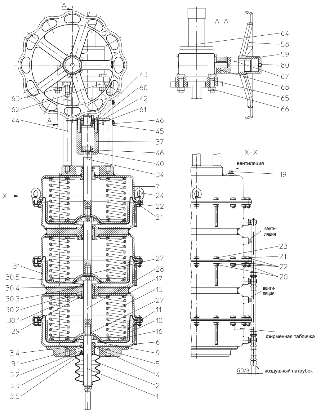
Рис. 6: DP34Tri шпindel привода выдвигается за счет силы пружины” с аварийным ручным управлением
