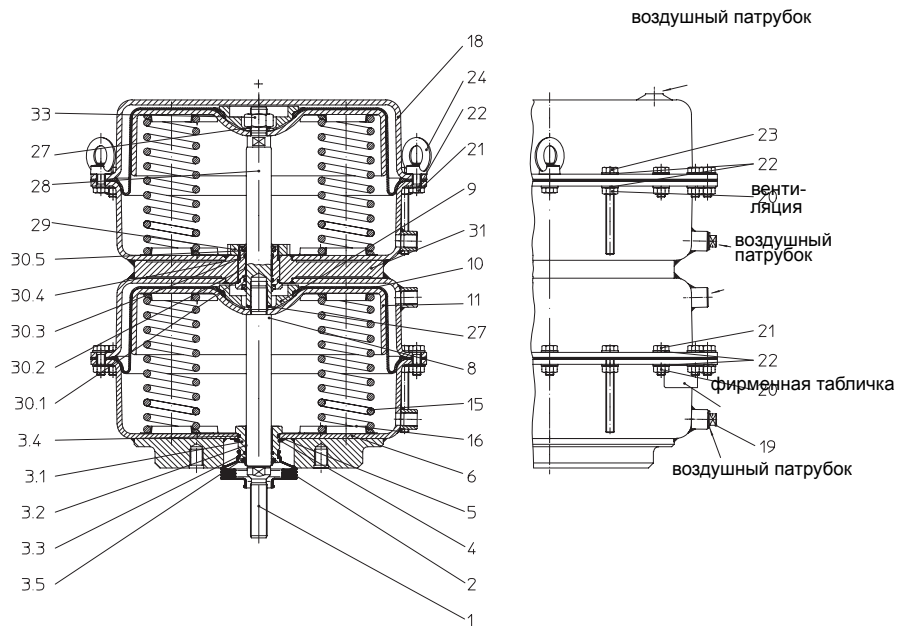
Рис. 3: DP34T „шпindelь привода втягивается за счет силы пружины“
