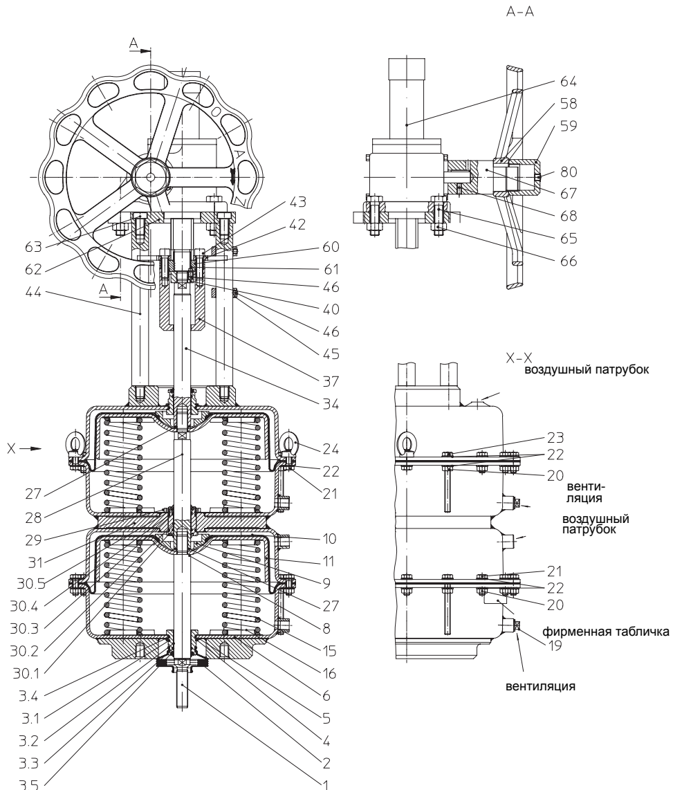
Рис. 4: DP34T „шпindelь привода втягивается за счет силы пружины“ с аварийным ручным управлением
