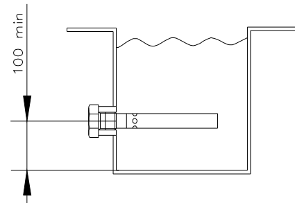
Рис 3 монтаж одиночного инжектора
