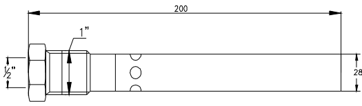
Рис 1 Основные размеры
