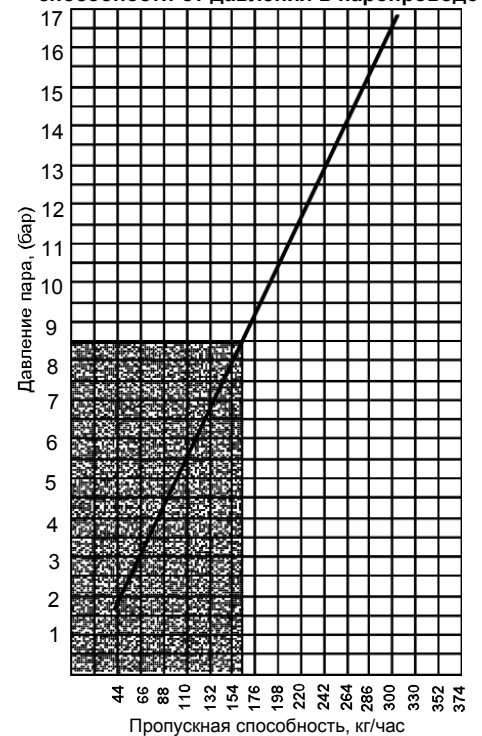
График зависимости пропускной способности от давления в паропроводе
